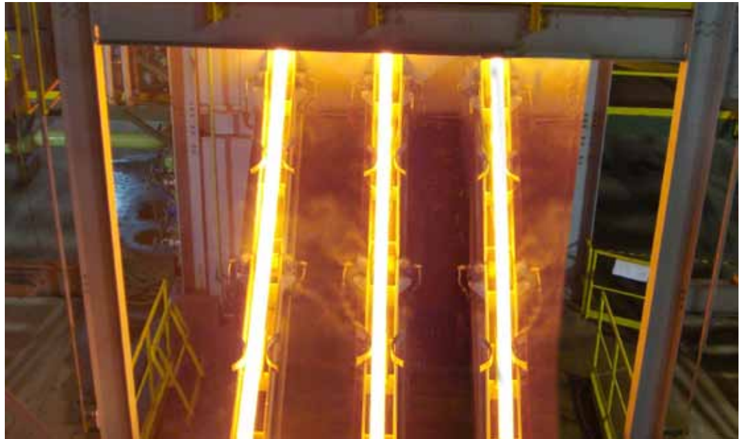
Lingotamento contínuo, um dos processos realizados na Aciaria
